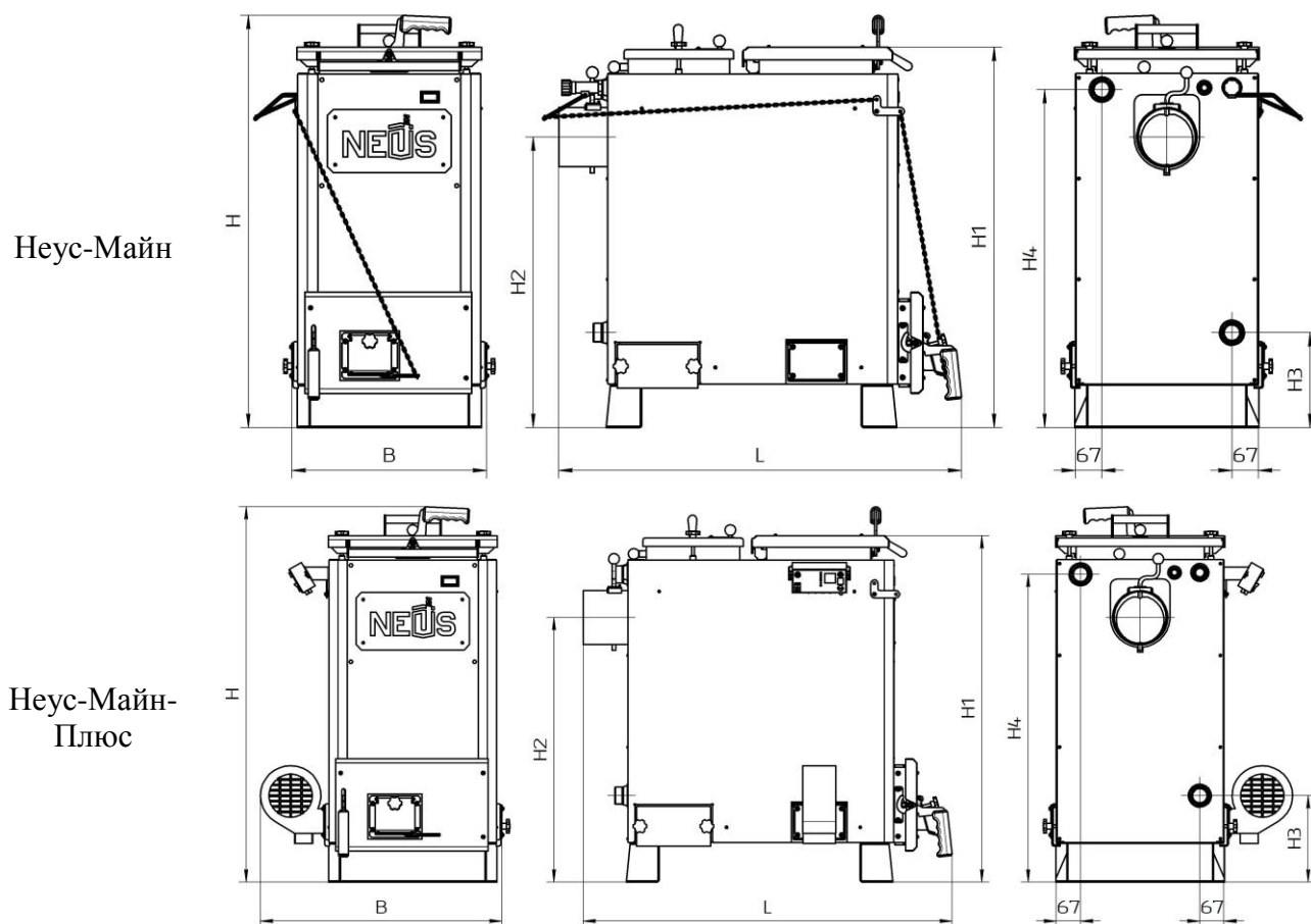
Рисунок 1 – Габаритне креслення котла Неус-Майн (Неус-Майн-Плюс)
