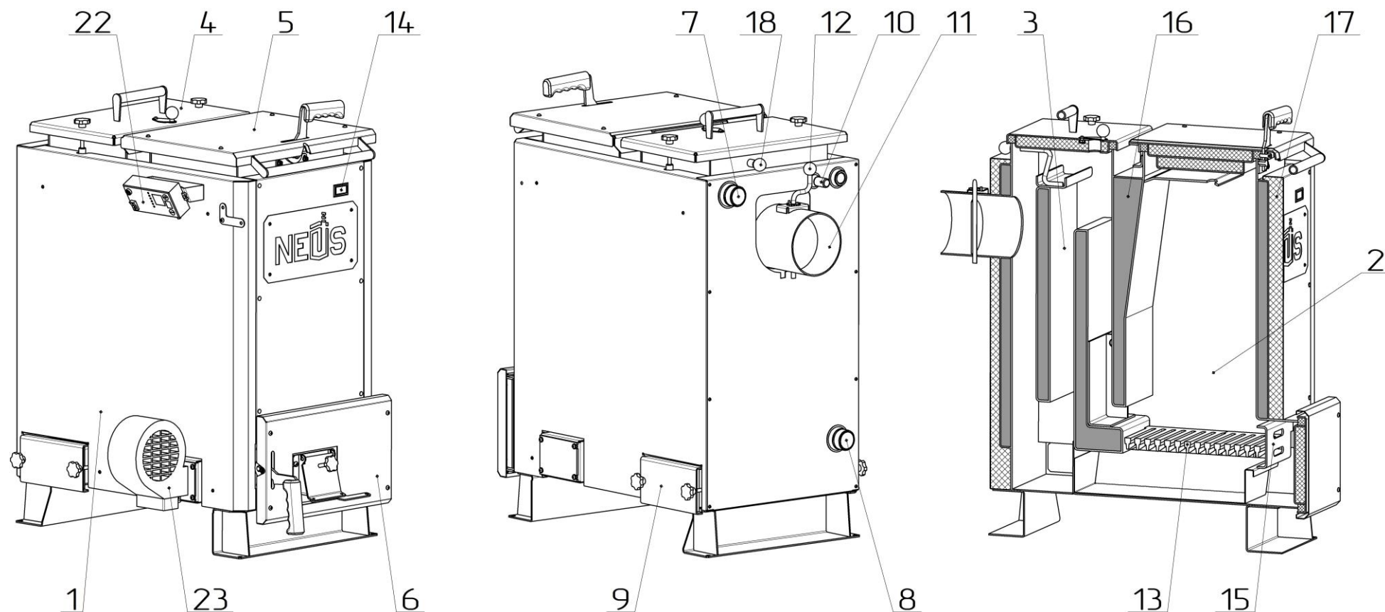
Рисунок 2б – Основні елементи котла Неус-Майн-Плюс
