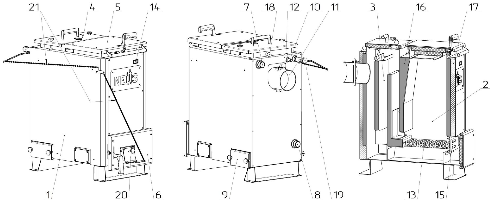
Рисунок 2а – Основні елементи котла Неус-Майн
